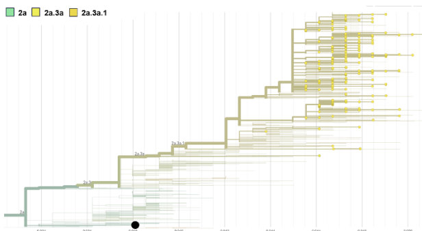
Fig. 8. Stamboom voor het hemagglutinine gen van A(H3N2) virussen. De gekleurde stippen geven Nederlandse virussen weer. De zwarte stip markeert de huidige vaccinstam. Dunne lijntjes representeren veelal oudere virussen van elders in de wereld. Clades zijn weergegeven in kleuren. De Nederlandse A(H3N2) virussen vallen in Clades 2a.3a en 2a.3a.1. Bron: Nextstrain, met dank aan GISAID.
